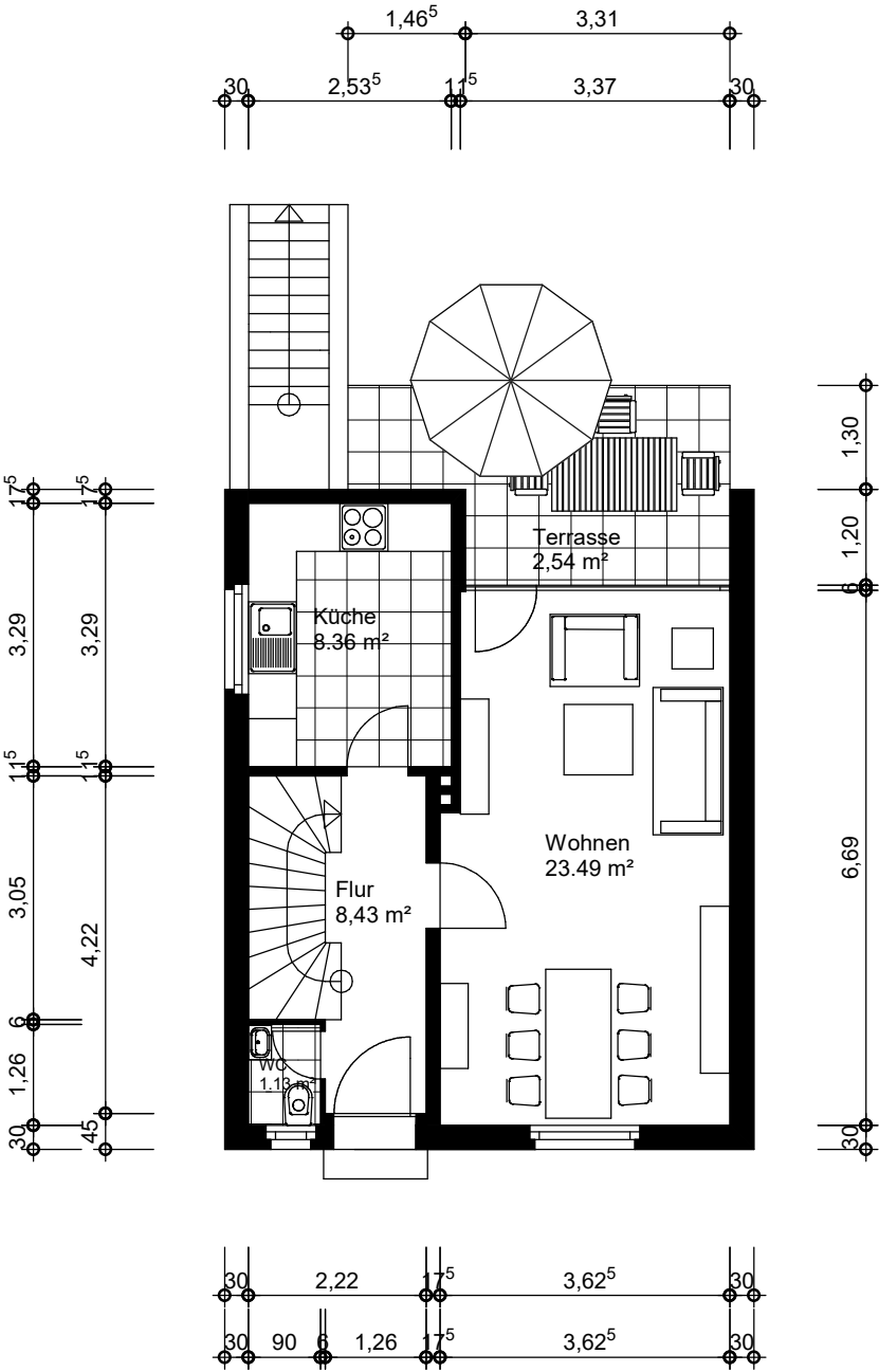
Erdgeschoss
